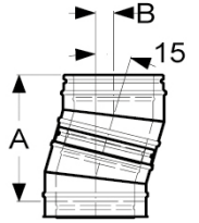
Afb. Bocht 30°
